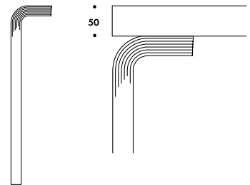
L-jalka 83LG on käytössä 5 cm paksuissa Aalto-pöydissä
